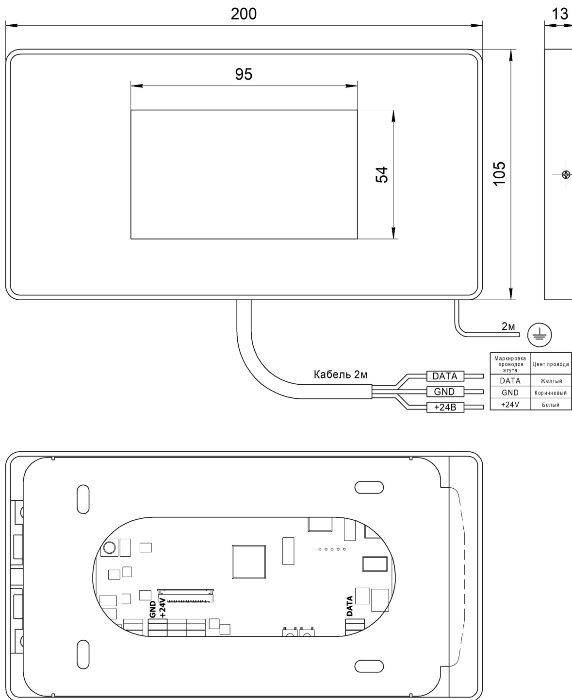
Рис.1 Внешний вид Табло накладное МАЛАХИТ НШЕК.468232.127-01 (дисплей 4,3)
